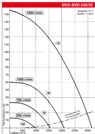
Figur 3. Exempel på ett kapacitetsdiagram för en brandgasfläkt. Vid 8 \text{ m}^3/\text{s} ( 28\,800 \text{ m}^3/\text{h} ), ett flöde vid öppna dörrar, kan den generera ca 250 Pa. Vid en halvering av flödet genom att dörrar stängs kan den generera över 1100 Pa.
