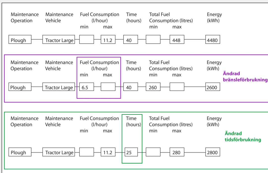
Figur 2. Exempel på hur modellen kan modifieras för att beräkna potentiella förändringar inom driften.
